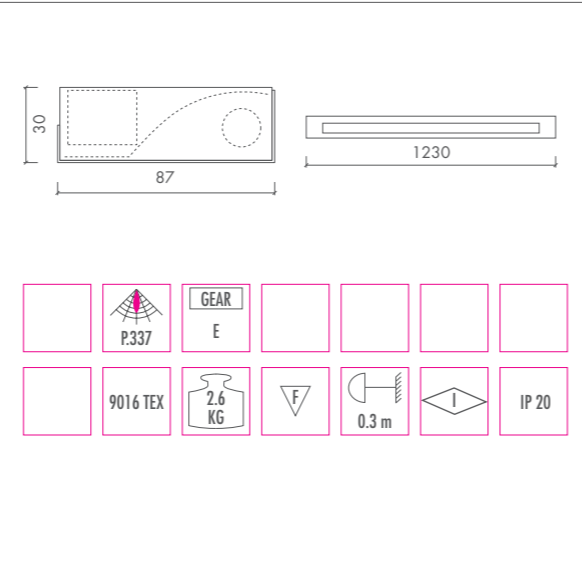
TASYM • T5 50W / 54W • G5
