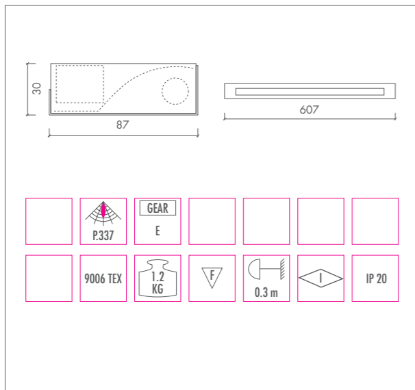
TASYM • T5 22W / 24W • G5
