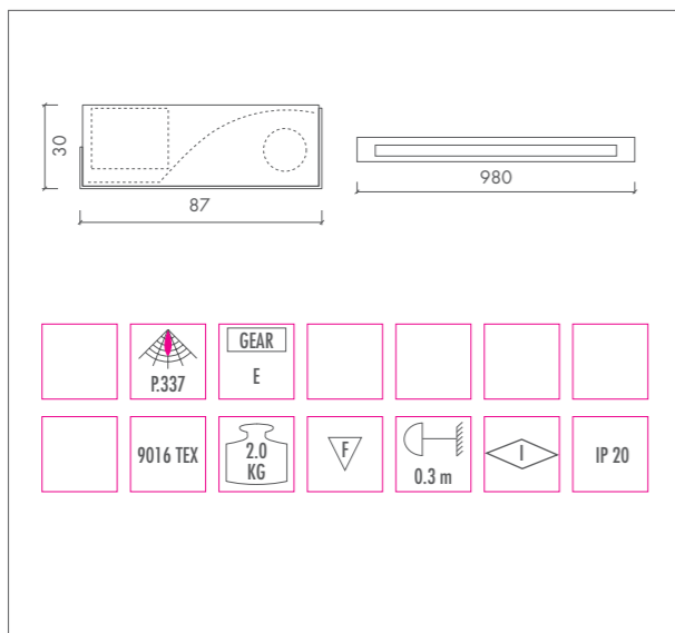
TASYM • T5 36W / 39W • G5
