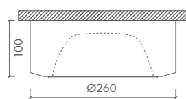
ECO UP 260 • TC-DE 2x18W • G24q2
