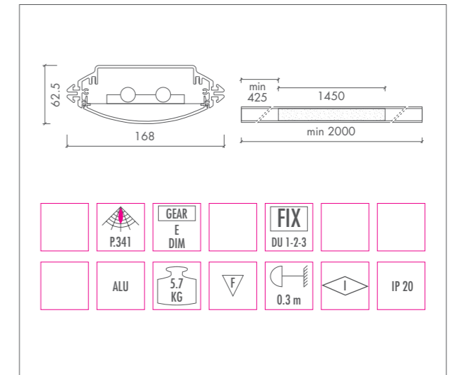
DUALIS T5 PLEXI • 2xT5 ECO 32W / 45W / 73W • 2xT5 35W / 49W / 80W • G5
