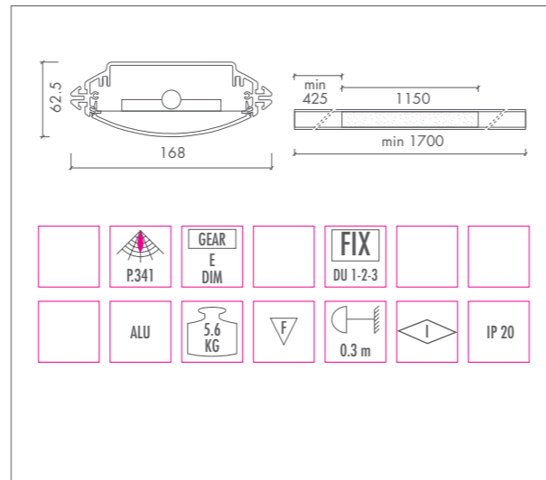
DUALIS T5 PLEXI • T5 ECO 25W / 50W • T5 28W / 54W • G5
