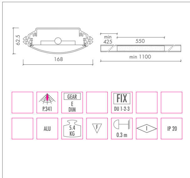
DUALIS T5 PLEXI • T5 14W / 24W • G5
