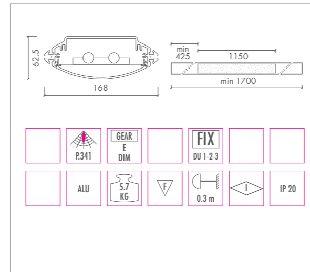
DUALIS T5 PLEXI • 2xT5 ECO 25W / 50W • 2xT5 28W / 54W • G5
