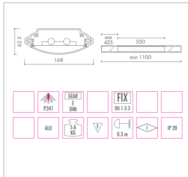
DUALIS T5 PLEXI • 2xT5 14W / 24W • G5
