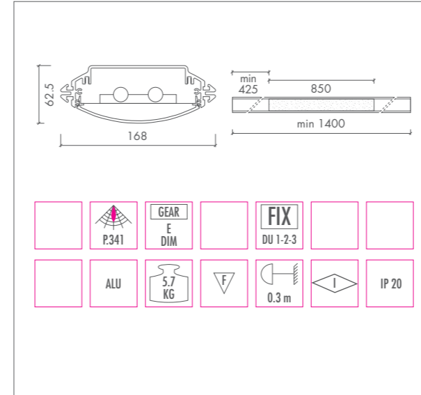
DUALIS T5 PLEXI • 2xT5 21W / 39W • G5
