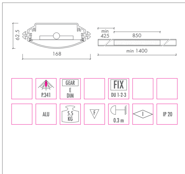
DUALIS T5 PLEXI • T5 21W / 39W • G5
