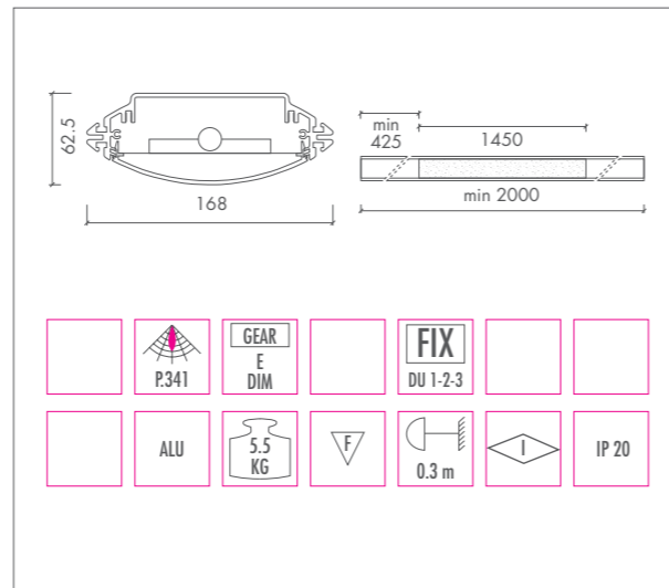
DUALIS T5 PLEXI • T5 ECO 32W / 45W / 73W • T5 35W / 49W / 80W • G5
