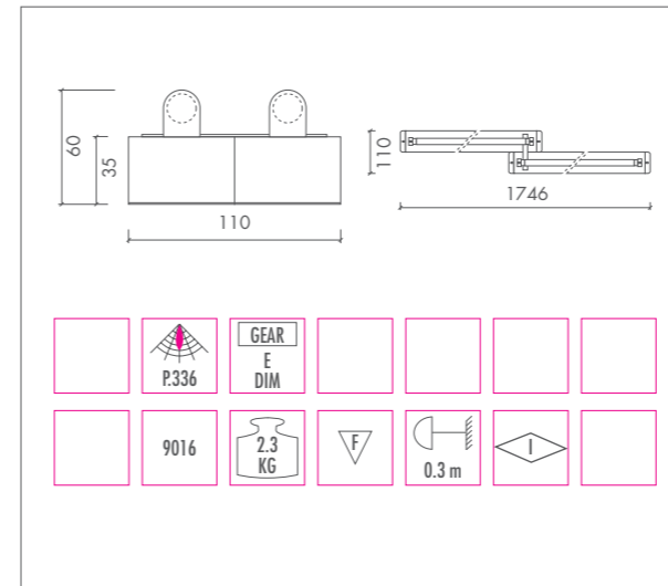
CROSS-LINE • 2xT5 19W / 21W / 36W / 39W • G5
