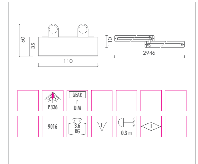
CROSS-LINE • 2xT5 32W / 35W / 45W / 49W / 73W / 80W • G5
