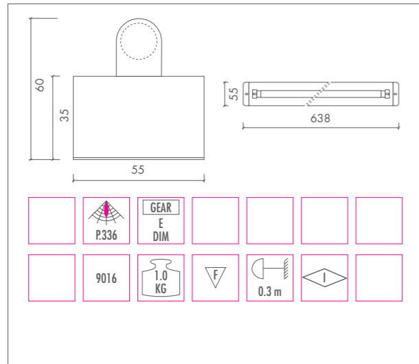
CROSS-LINE • 1xT5 13W / 14W / 22W / 24W • G5
