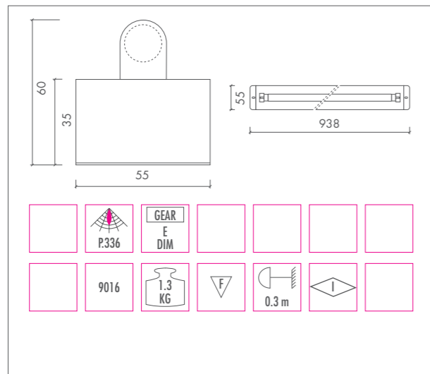
CROSS-LINE • 1xT5 19W / 21W / 36W / 39W • G5
