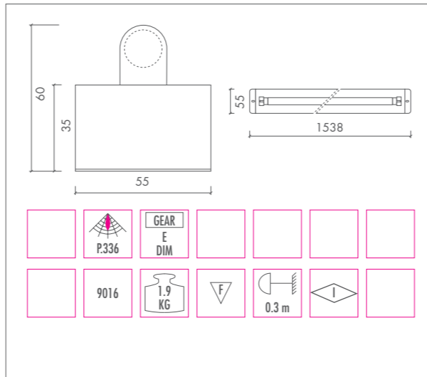
CROSS-LINE • 1xT5 32W / 35W / 45W / 49W / 73W / 80W • G5
